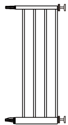
Extensión de 4 barras 9.89" (25.1 cm)
